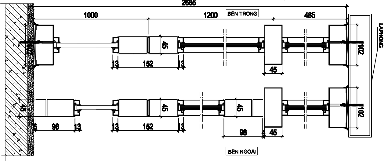
MẶT CẮT: 1-1 TTL: 1/4
